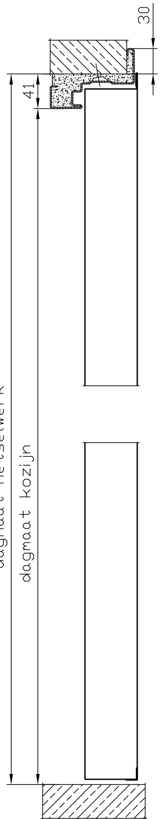
Doorsnede B-B
