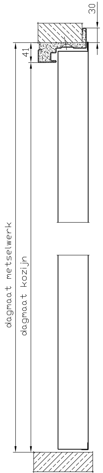
Doorsnede B-B
