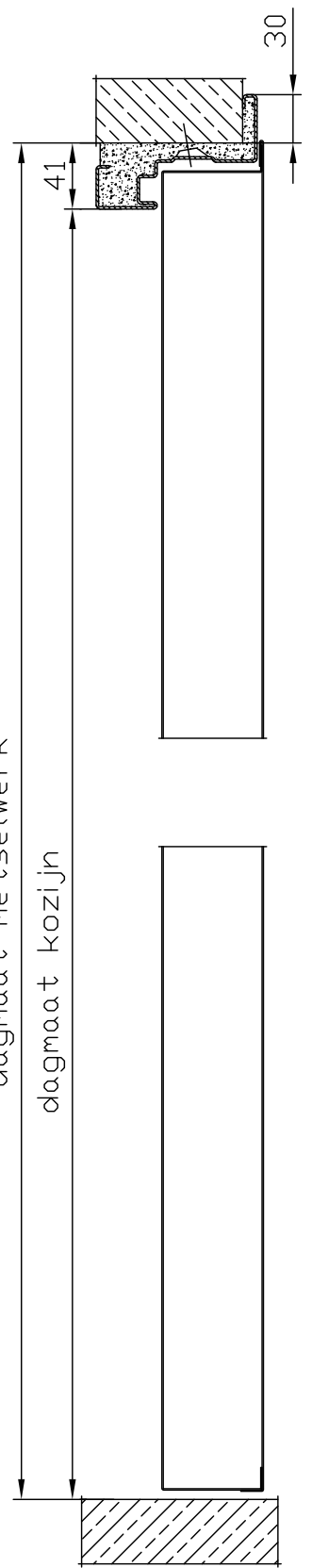
Doorsnede B-B
