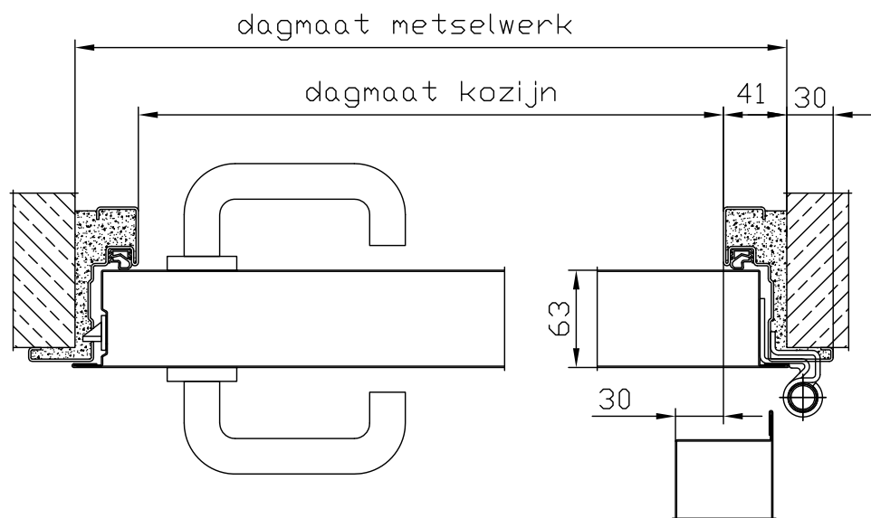
Doorsnede A-A
