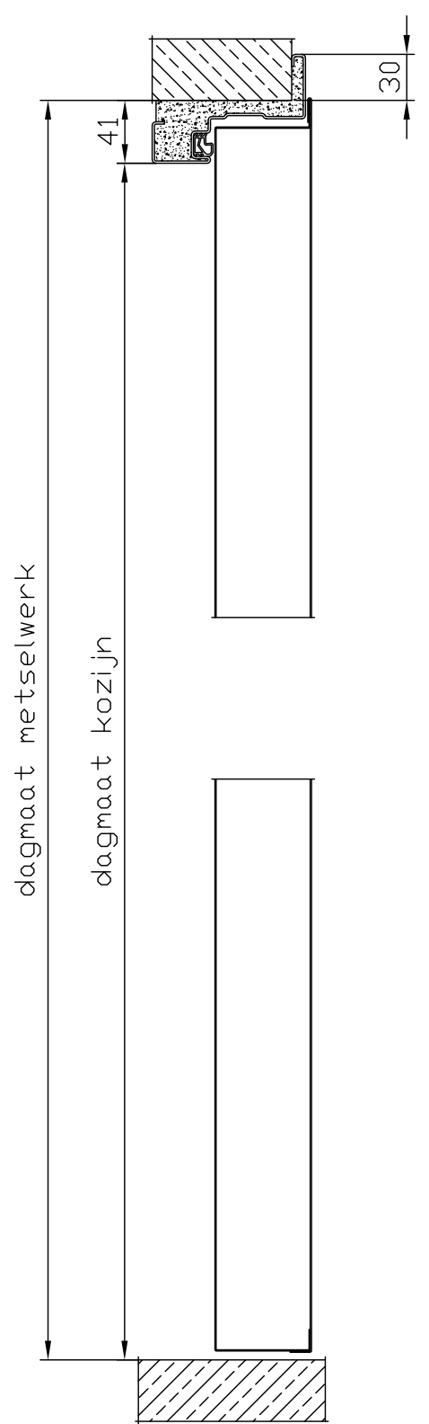
Doorsnede B-B
